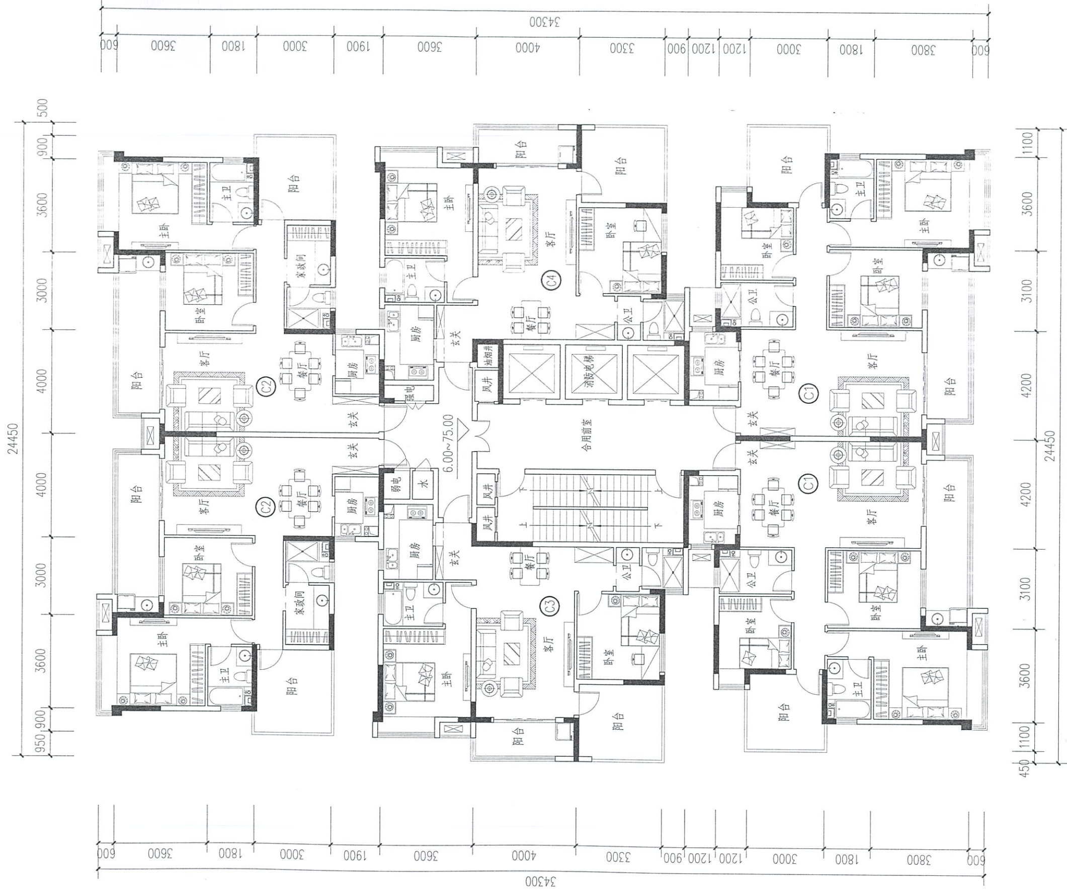
9#楼三至二十六层平面图 1:100
